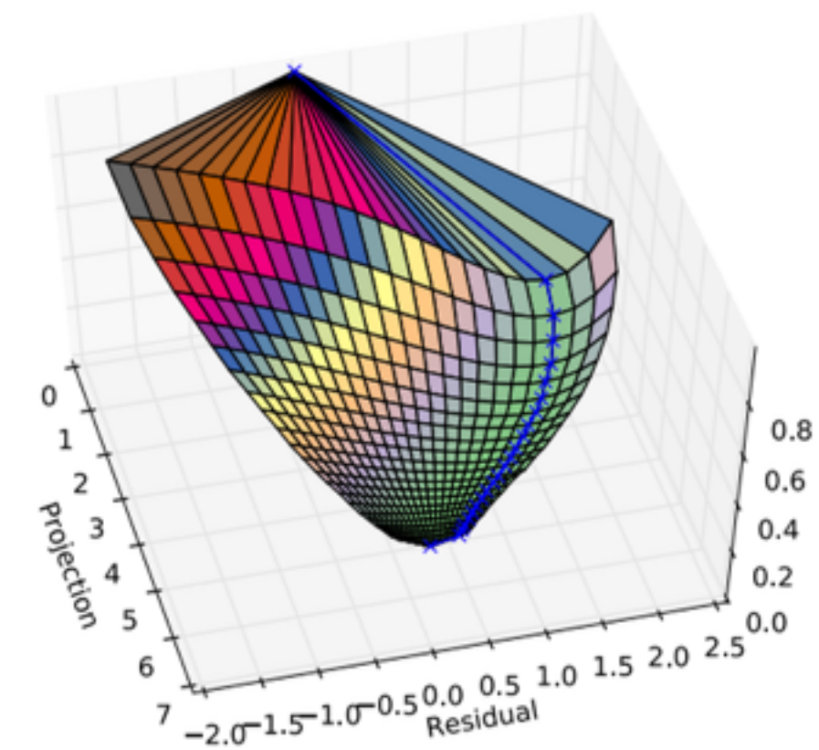
Factored Linear
